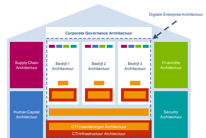
Figuur 3: Voorbeeld van een generiek Dragon1 architectuurraamwerk dat u kunt aanpassen aan uw eigen situatie.
